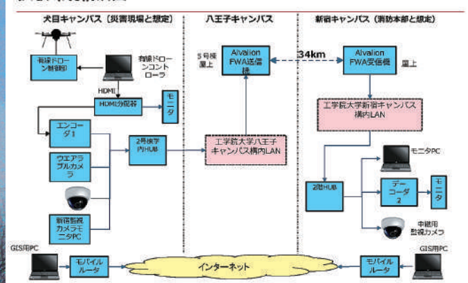
試験環境構成図
